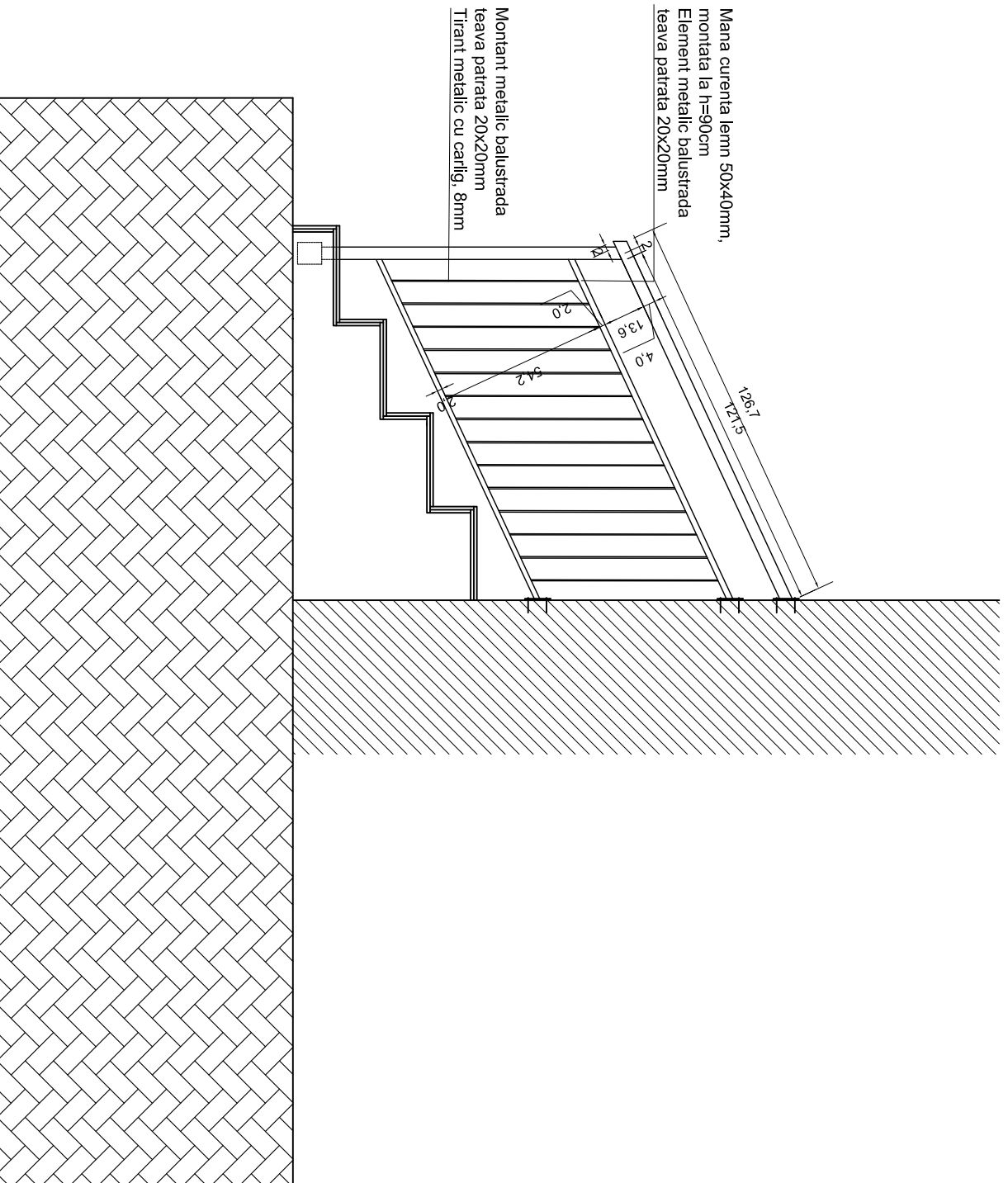
VEDERE SCARA - MANA CURENTA SC. 1:50
